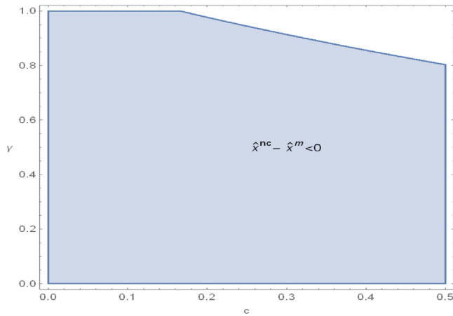
Fig. 1. \hat{x}^{nc} < (>)\hat{x}^m .
